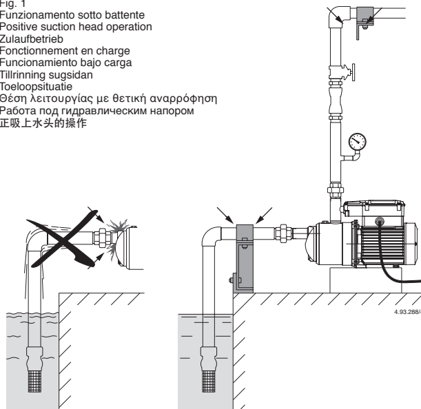
Fig. 2 Funzionamento in aspirazione Suction lift operation Saugbetrieb Fonctionnement en aspiration Funcionamiento en aspiración Sugande funktion Zuigsituatie Θέση λειτουργίας με κάθετη αναρρόφηση Работа выше уровня жидкости 负压吸水头工作
