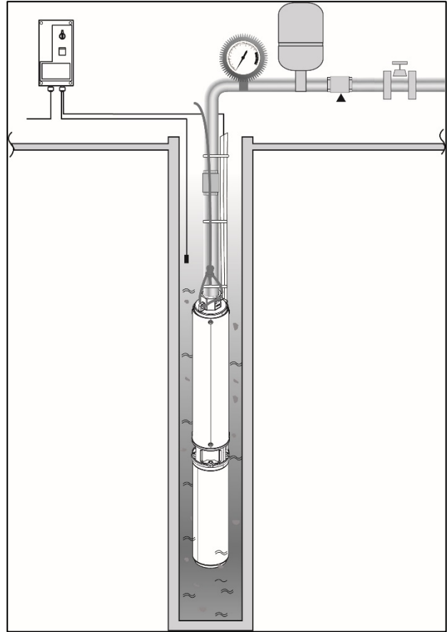
Şek.2 Kurma örneği
