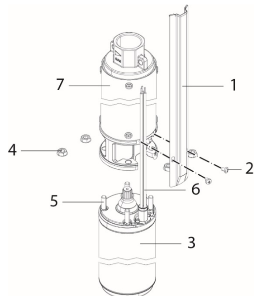
1. ábra Motor-pumpa csatlakoztatás
