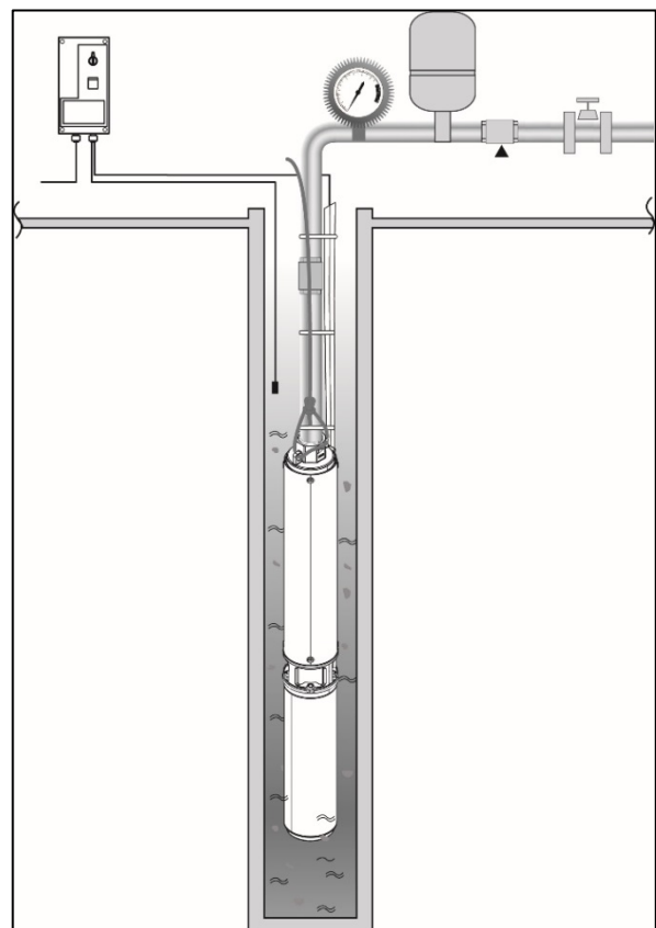
Abb. 2 Installationsbeispiel
