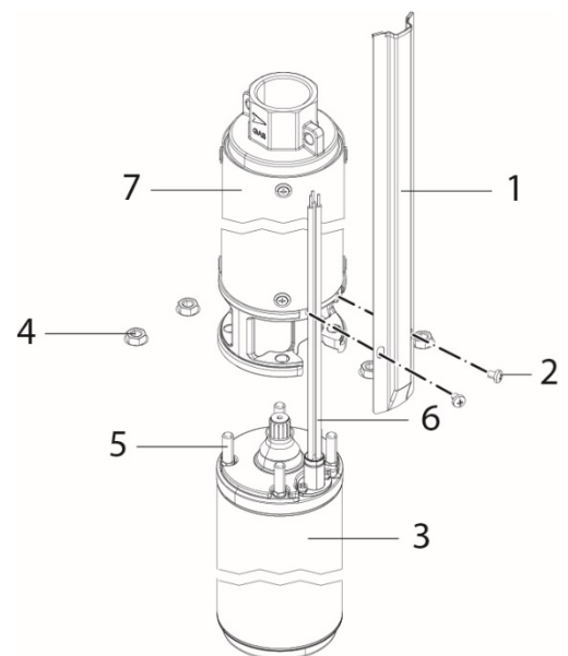
Image 1 Couplage pompe-moteur
