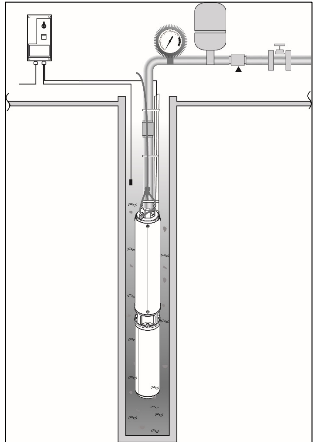
Fig.2 Exemplo de instalação
