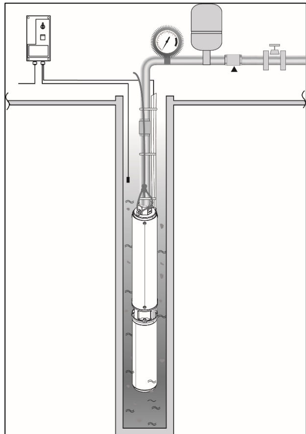
Obr.2 Příklad instalace
