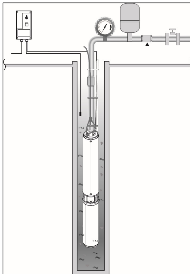
Fig.2 Пример за инсталиране
