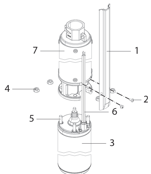
Abb. 1 Kopplung Pumpe-Motor
