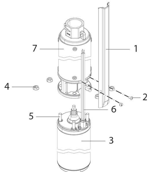
Obr. 1 Sestava čerpadlo-motor
