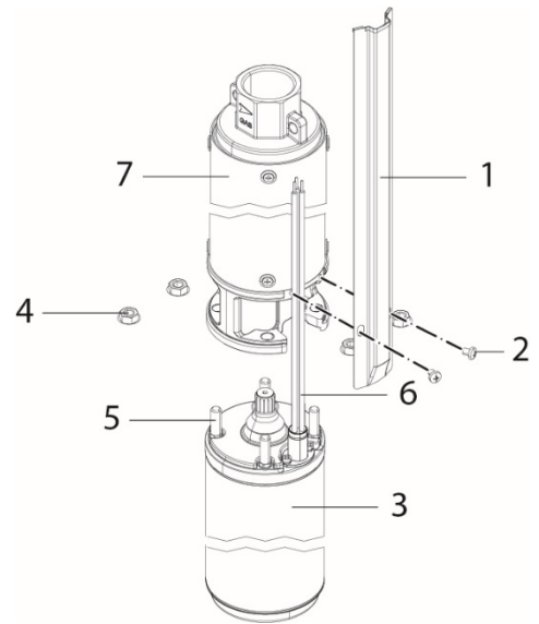
Fig. 1 Accoppiamento pompa-motore
