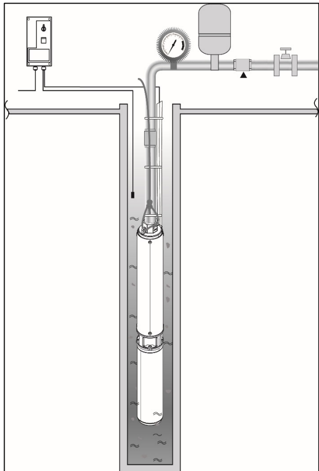
Рис. 2 Пример монтажа
