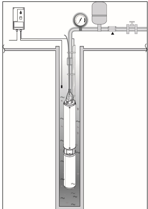
2. ábra Beszerelési példa
