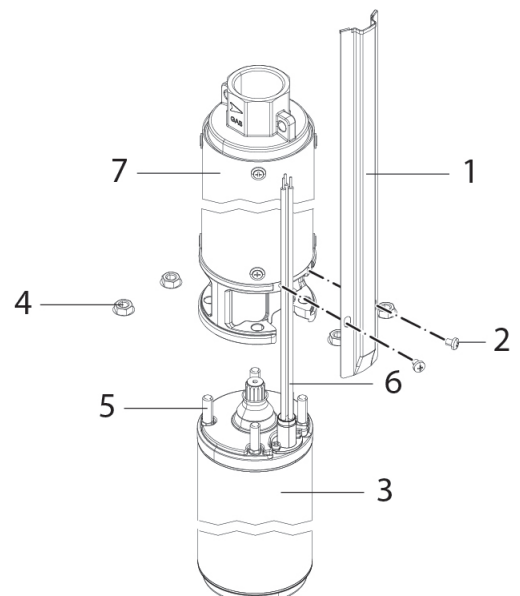
Rys. 1 Połączenie pompa-silnik
