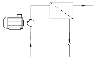
Fig. 20 Module de surpression BME - sens du nettoyage
