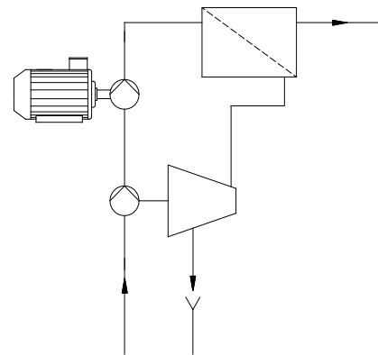
Fig. 21 Module de surpression BMET - sens du nettoyage
