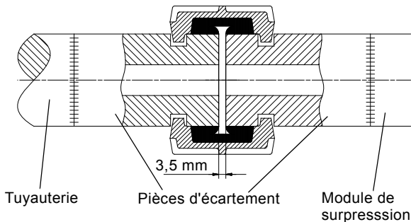
Fig. 8 Position des pièces d'écartement
