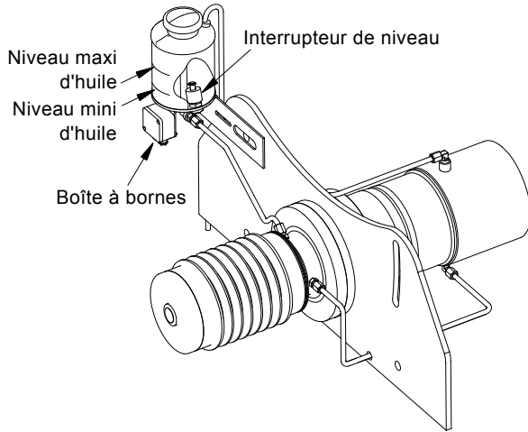
Fig. 10 Système de lubrification à l'huile
