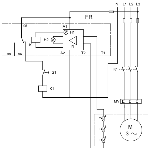
Fig. 9 Schéma de câblage
