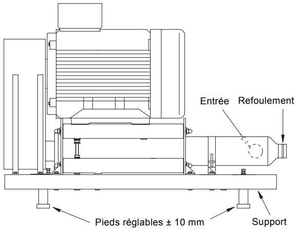
Fig. 3 Module de surpression BME
