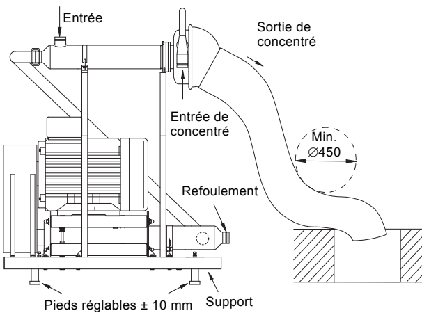
Fig. 4 Module de surpression BMET
