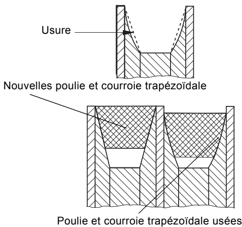
Fig. 13 Exemples de poulies cannelées usées et nouvelles
