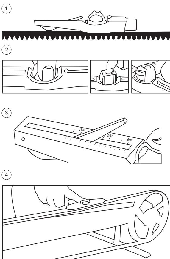
Fig. 16 Contrôleur de tension
