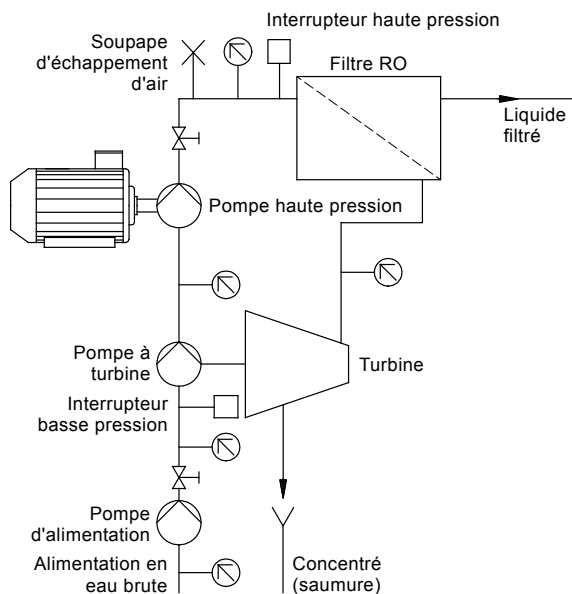
Fig. 12 Système de surpression BMET
