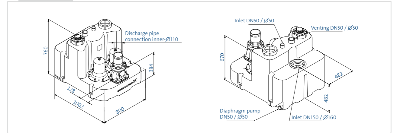
MULTILIFT MLD
