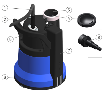
Simer 6S z wyłącznikiem zanurzeniowym
