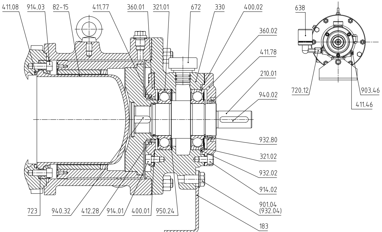
III. 15: Version support de palier lubrifié à l'huile sans bague d'étanchéité d'arbre faisant office de barrière de fuite
