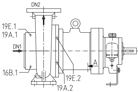
III. 7: Raccords pour le réchauffage 14)
