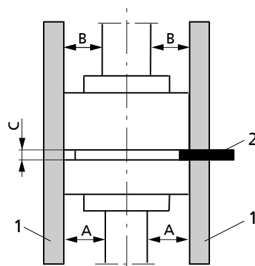
III. 3: Contrôler le lignage de l'accouplement
