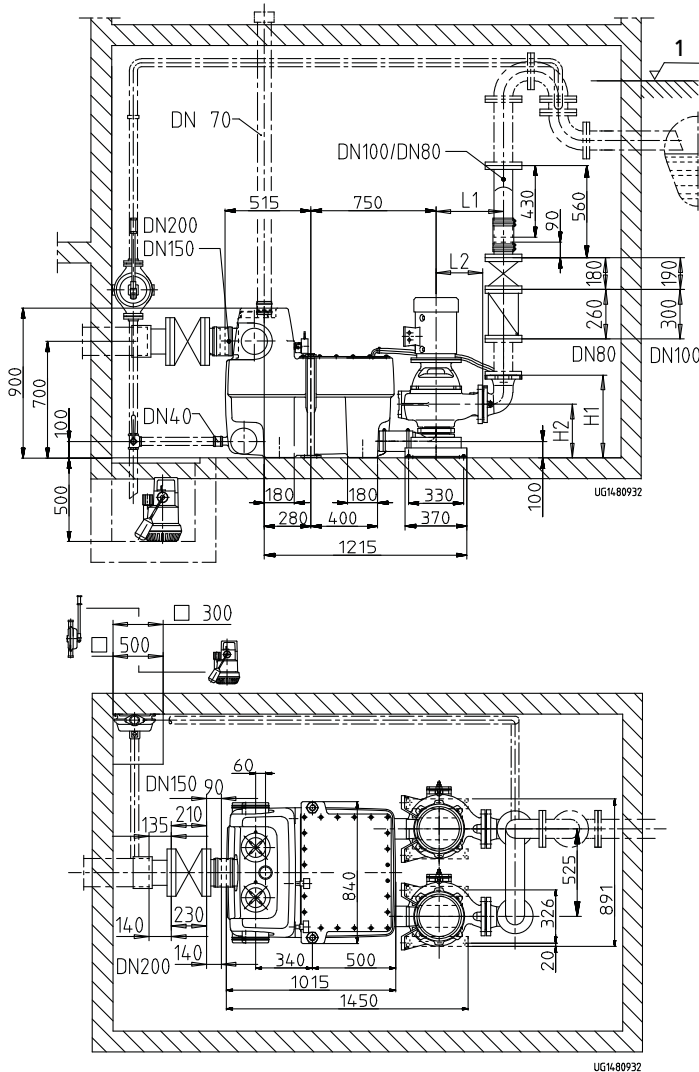
Cotes d'installation Compacta UZ, ZF, ZK .. 450 D [mm]
