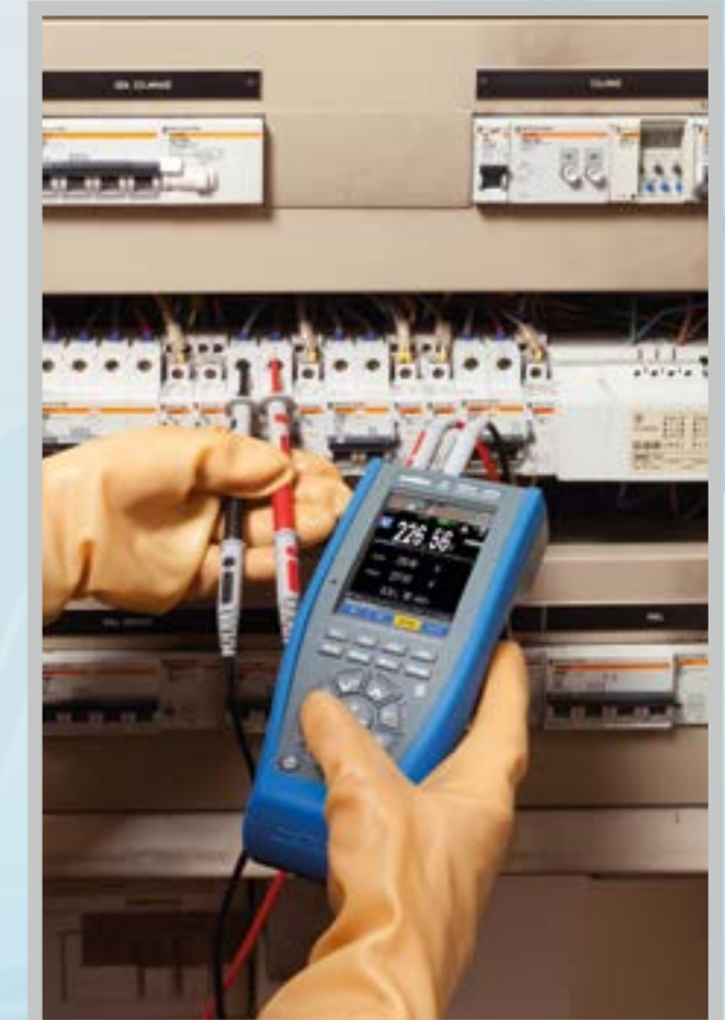
Mesures sur armoires électriques
