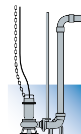
Avec DISPOSITIF D'ACCOUPLAGE SUR LE FOND
